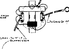
157 I.F. INPUT TRANSFORMER R7725A
